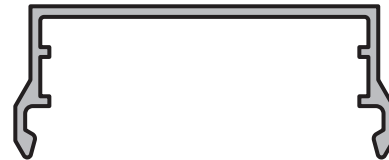
TAPA DE LARGUERO Perfil: 2636 Peso: 0,343 Kg/m
