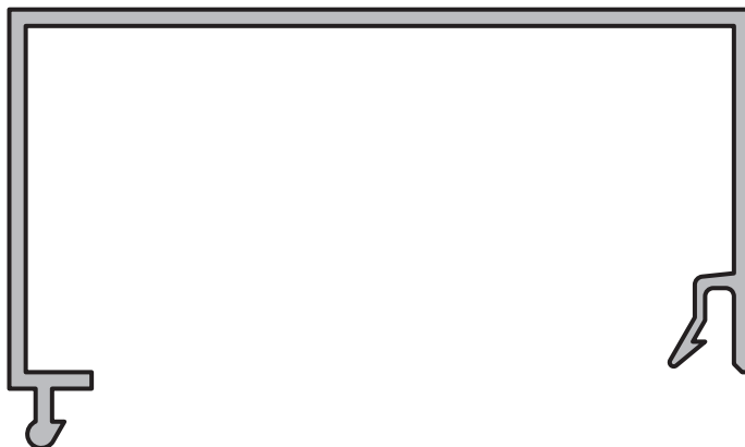
SEMITUBO PARA CUADRADO DE 90 x 90 mm. Perfil: 2719 Peso: 1,104 Kg/m
