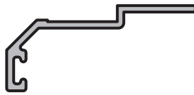
MARCO DE PUERTA Perfil: 191 Peso: 0,178 Kg/m Matriz: M2550
