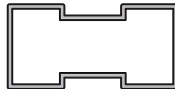
TRAVESAÑO Perfil: 194 Peso: 0,464 Kg/m Matriz: M2553
