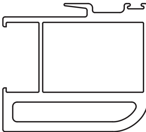
PERFIL 6087 2,816 kg/m
