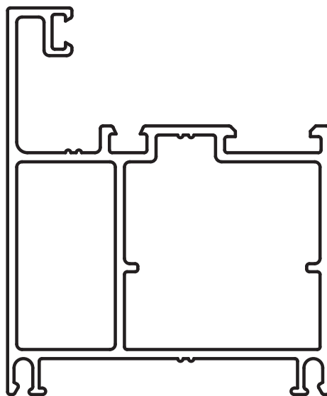
PERFIL 7656 1,507 kg/m
