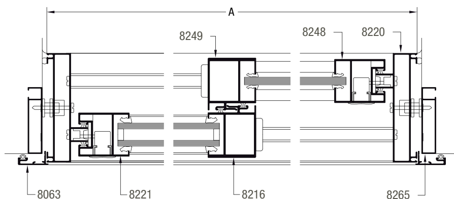
SECCION 1-2-3
