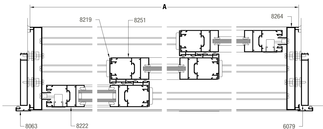
SECCION 12-13-14-15
