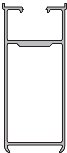
BATIENTE SIN CONTRAVIDRIOS Perfil: 6350 Peso: 0,977 Kg/m
