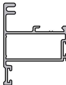
HOJA VENTILUZ Perfil: 218 Peso: 0,548 Kg/m Matriz: M2707
