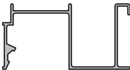
GUÍA CORTINA DE ENROLLAR Perfil: 920 Peso: 0,456 Kg/m Matriz: M2355
