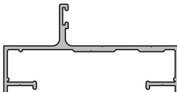
MARCO Perfil: 10 Peso: 0,788 Kg/m Matriz: M0676
