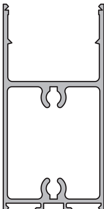
TRAVESAÑO HOJA Perfil: 11 Peso: 1,671 Kg/m Matriz: M0677
