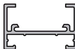
SOPORTE TABLILLA DE POSTIGON Perfil: 148 Peso: 0,340 Kg/m Matriz: M1986
