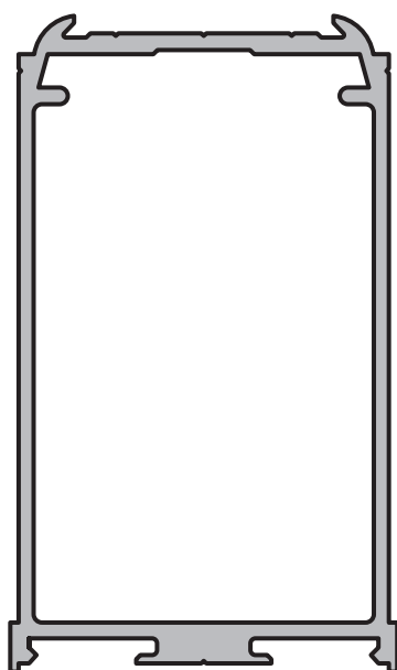
PARANTE HOJA Perfil: 39 Peso: 1,364 Kg/m Matriz: M0796
