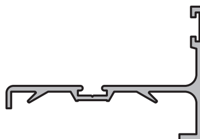
TAPACANTO CON TOPE PARA BATIENTE Perfil: 42 Peso: 0,481 Kg/m Matriz: M0799
