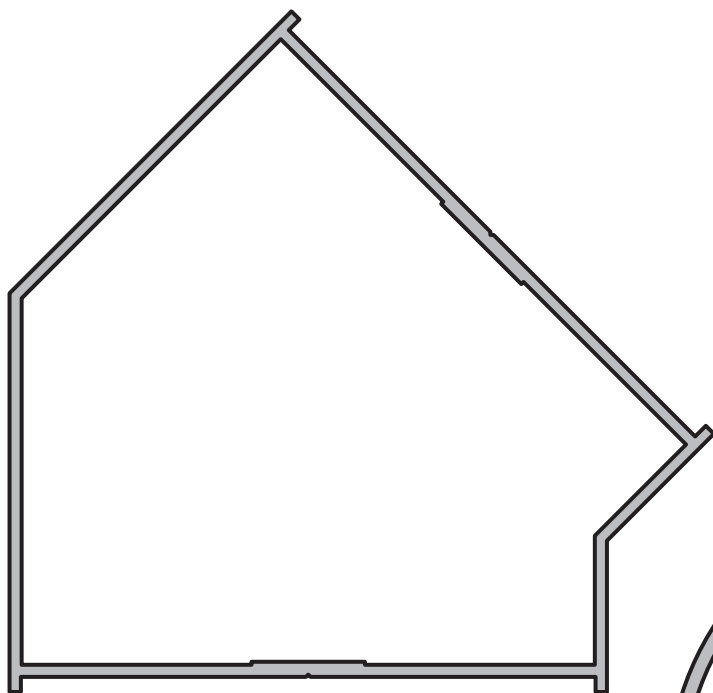
TUBO DE ACOPLE A 45 Perfil: 718 Peso: 1,320 Kg/m Matriz: M2506
