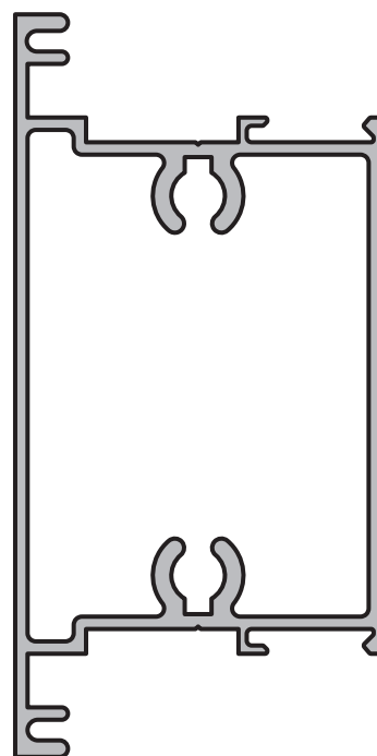
TRAVESAÑO INTERMEDIO Perfil: 208 Peso: 1,369 Kg/m Matriz: M2696
